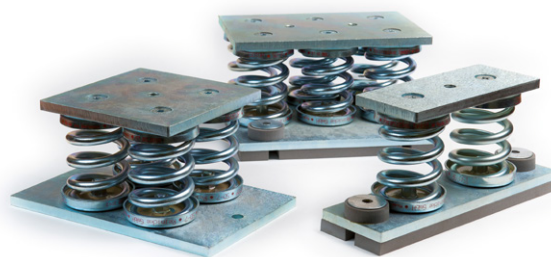
Vibrofix Spring SD (сблокированные)
